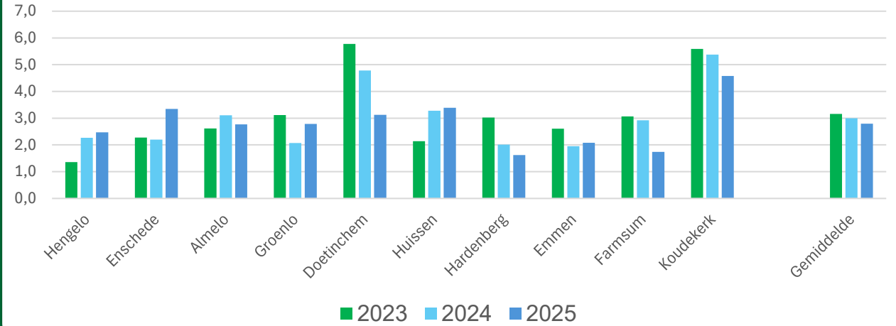
Betonggranulaat % per m3 t.o.v. totaal toeslagmateriaal
